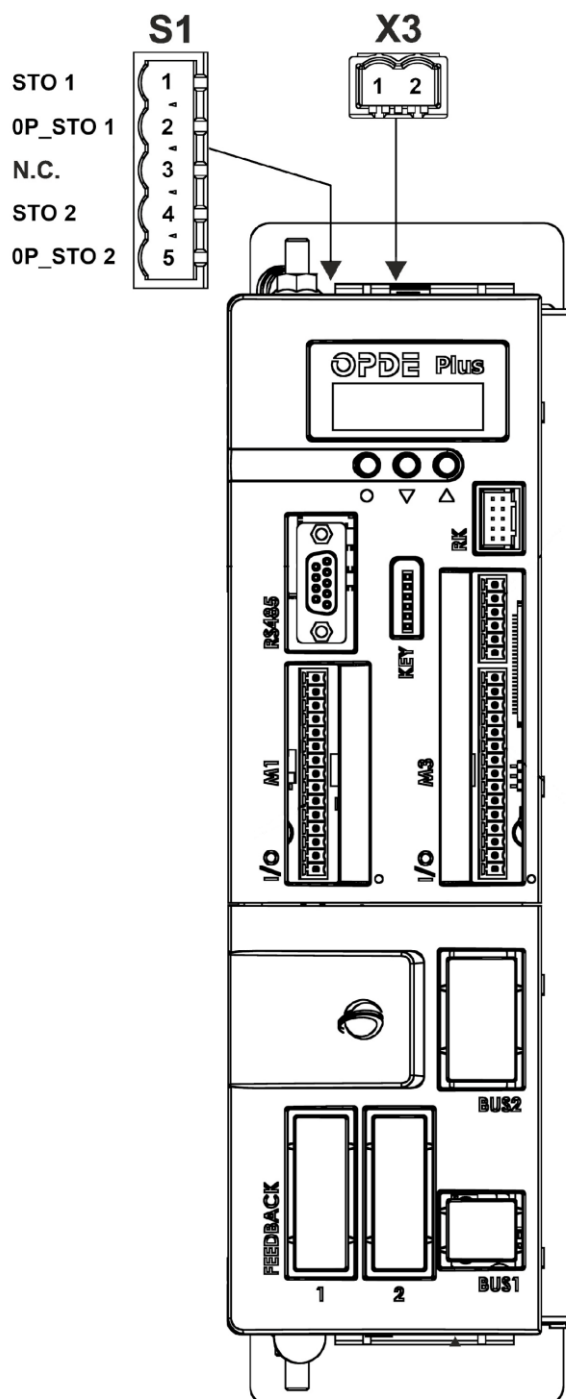
FIG. 2- Posizione dei connettori X3 e S1 / Position of terminals board X3 and S1
